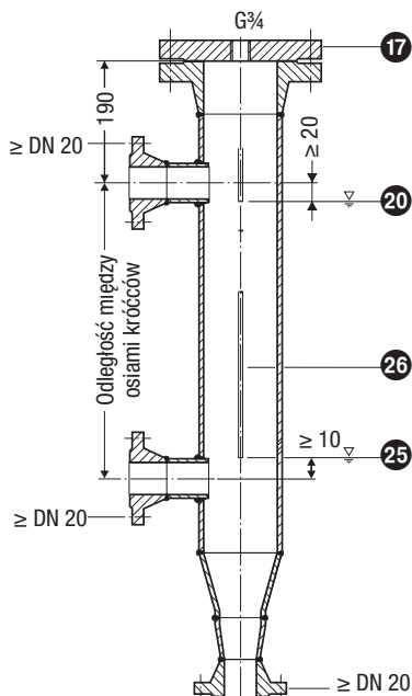
Rys. 18 Naczynie pomiarowe \geq DN 80 przy zastosowaniu elektrody jako zewnętrznego ogranicznika poziomu wody
