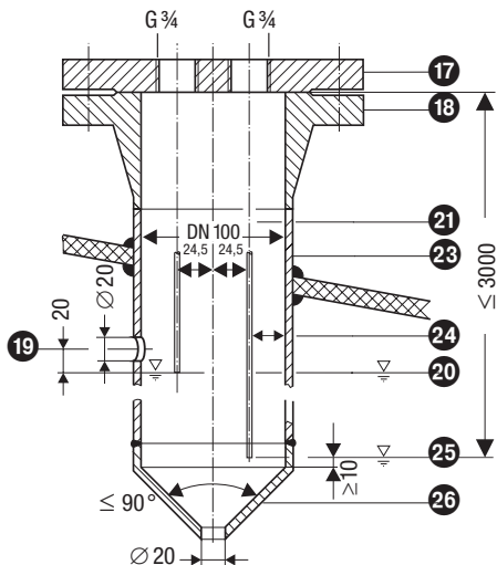
Rys. 17 Rura ochronna (nie jest przedmiotem dostawy) przy zastosowaniu elektrody jako wewnętrznego ogranicznika poziomu wody w połączeniu z regulatorem i zabezpieczeniem przed zbyt wysokim poziomem wody.
